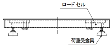
ロードセル 4点式 台秤 BAPシリーズ
