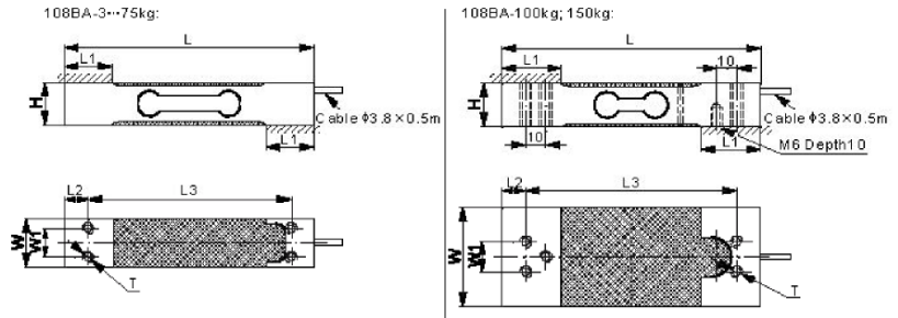
寸法図
