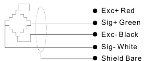
結線図
